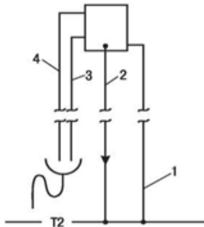
Рисунок 7 – Схема подключения расширительного бака в систему отопления
