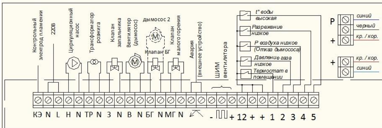
Рисунок 3 – Принципиальная электрическая схема
