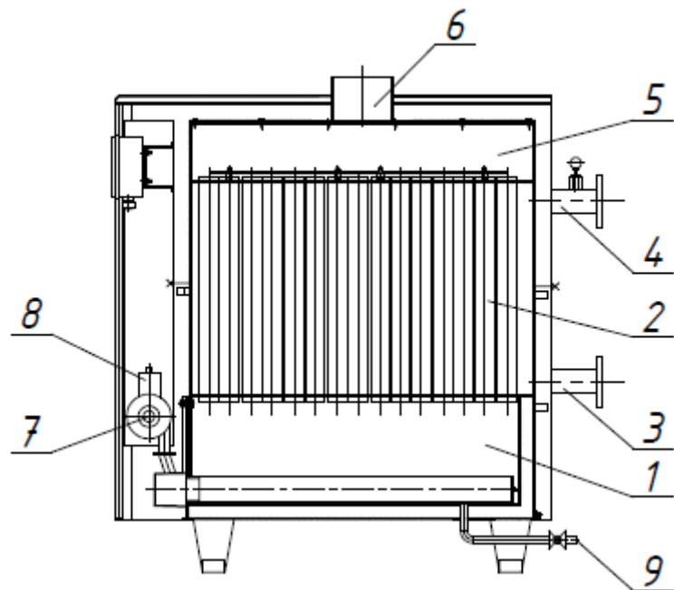
Рисунок 4 – Теплообменник котла
