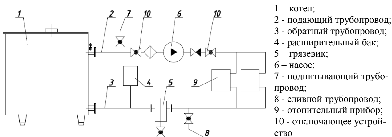
Рисунок 9 – Принципиальная схема системы отопления
