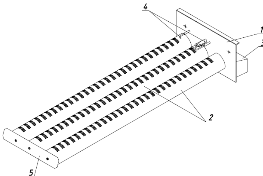
Рисунок 5 – Горелочное устройство котла
